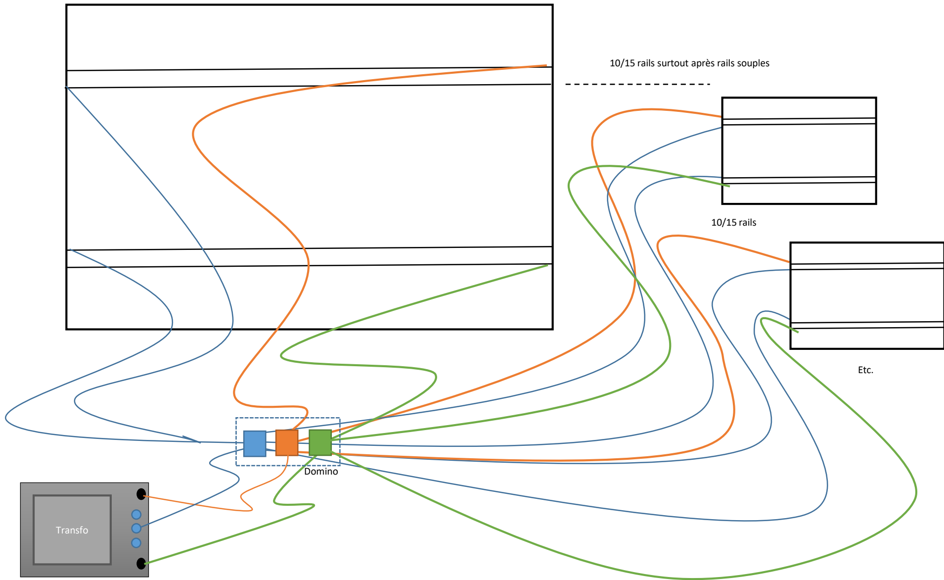
Araignée pour Circuit 24 24V alternatif
