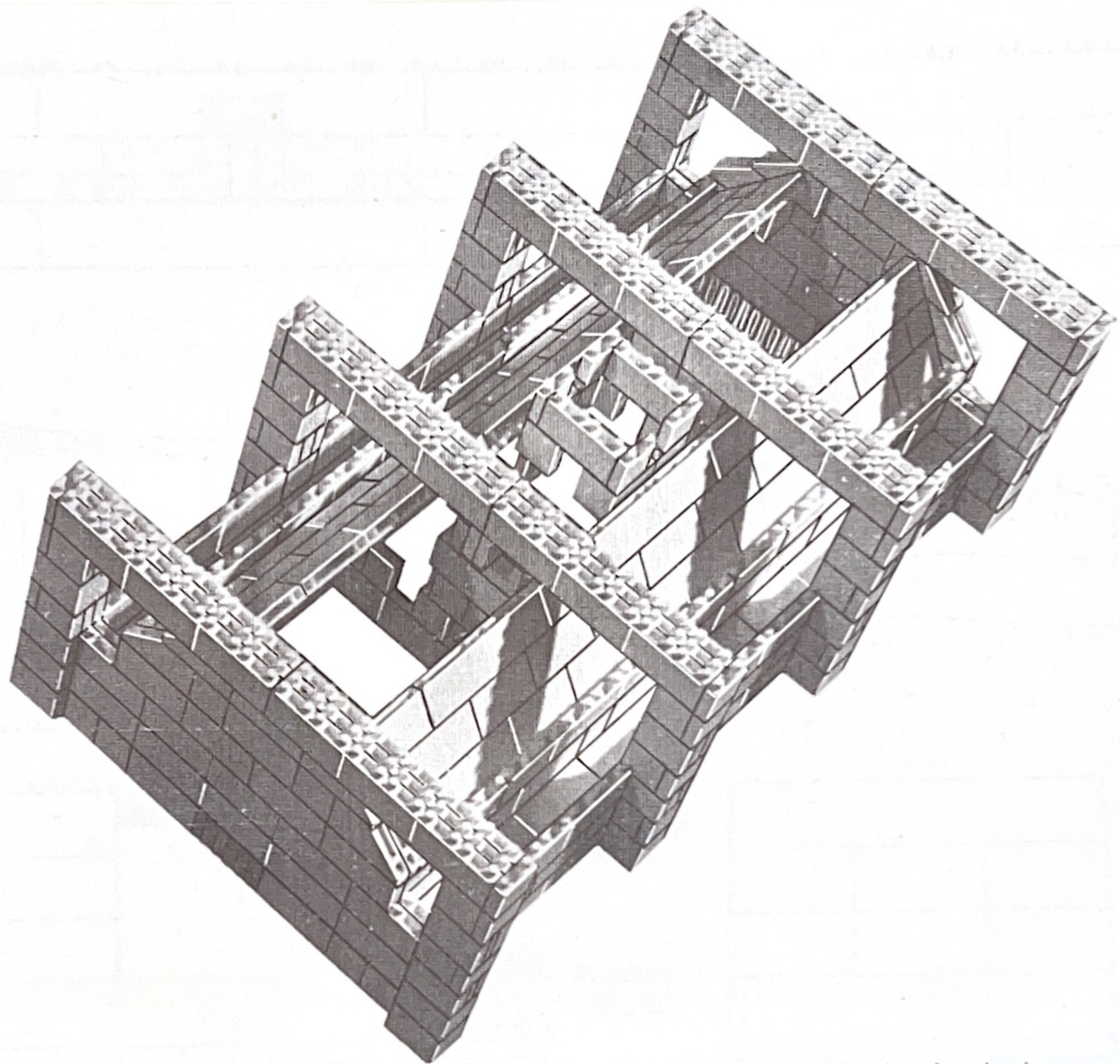
Cette photo montre comment monter les 2 toits inclinés, (construits selon le dessin de la page 20), les 4 grandes poutres et enfin la base de la flèche.
